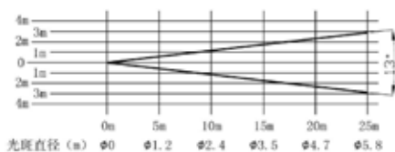
正焦最大光斑图
