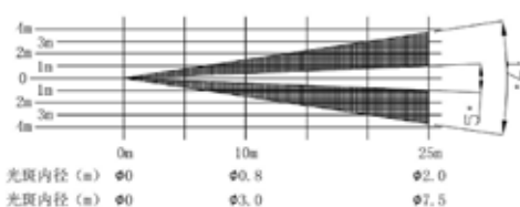
反焦最大光斑图
