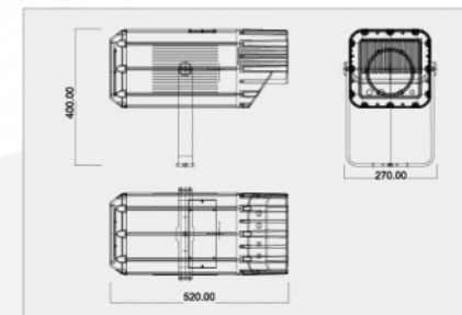
产品尺寸图
